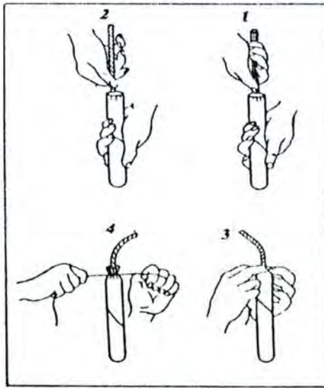
شکل ۵-۲- مراحل مختلف چاشنی گذاری
