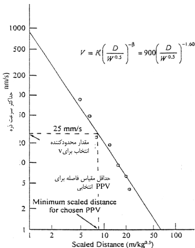
شکل ۹-۶- نمودار تغییرات ماکزیمم سرعت ذره ای نسبت به فاصله در مقیاس تمام لگاریتمی
